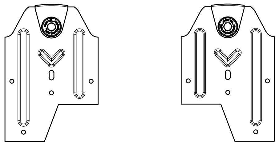
Monture gauche Left hanger Monture droite Right hanger
