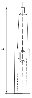
Cono interno-Internal Morse DIN 228
