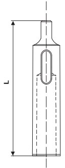
Cono interno-Internal Morse DIN 228
